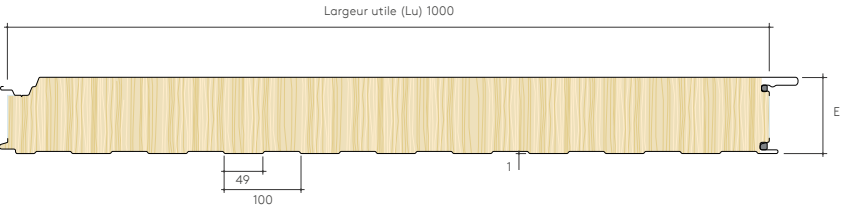
Profil lisse
