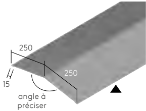
Sous-faîtière
