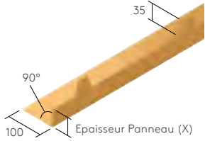
Closoir cranté
