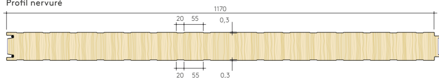
Profil nervuré
