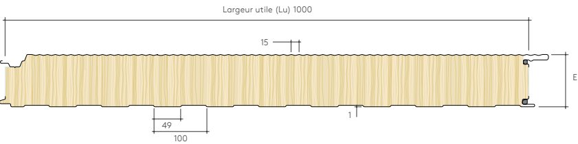
Profil micro-nervuré
