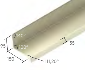
Rive contre mur
