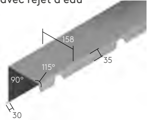
Bandeau de faîtage crantée avec rejet d'eau
