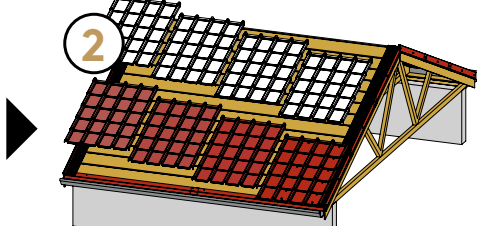
POSE DES TUILES DE BAS EN HAUT
