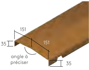
Faîtière double crantée
