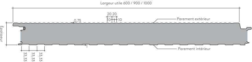
Profil Micro-Rib*
