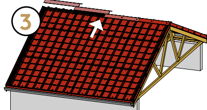
POSE DES FAÎTIÈRES
