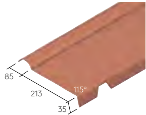
Demie faîtière à boudin
