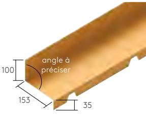
Faîtière contre mur crantée
