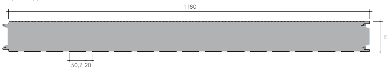
Profil Twinlook
