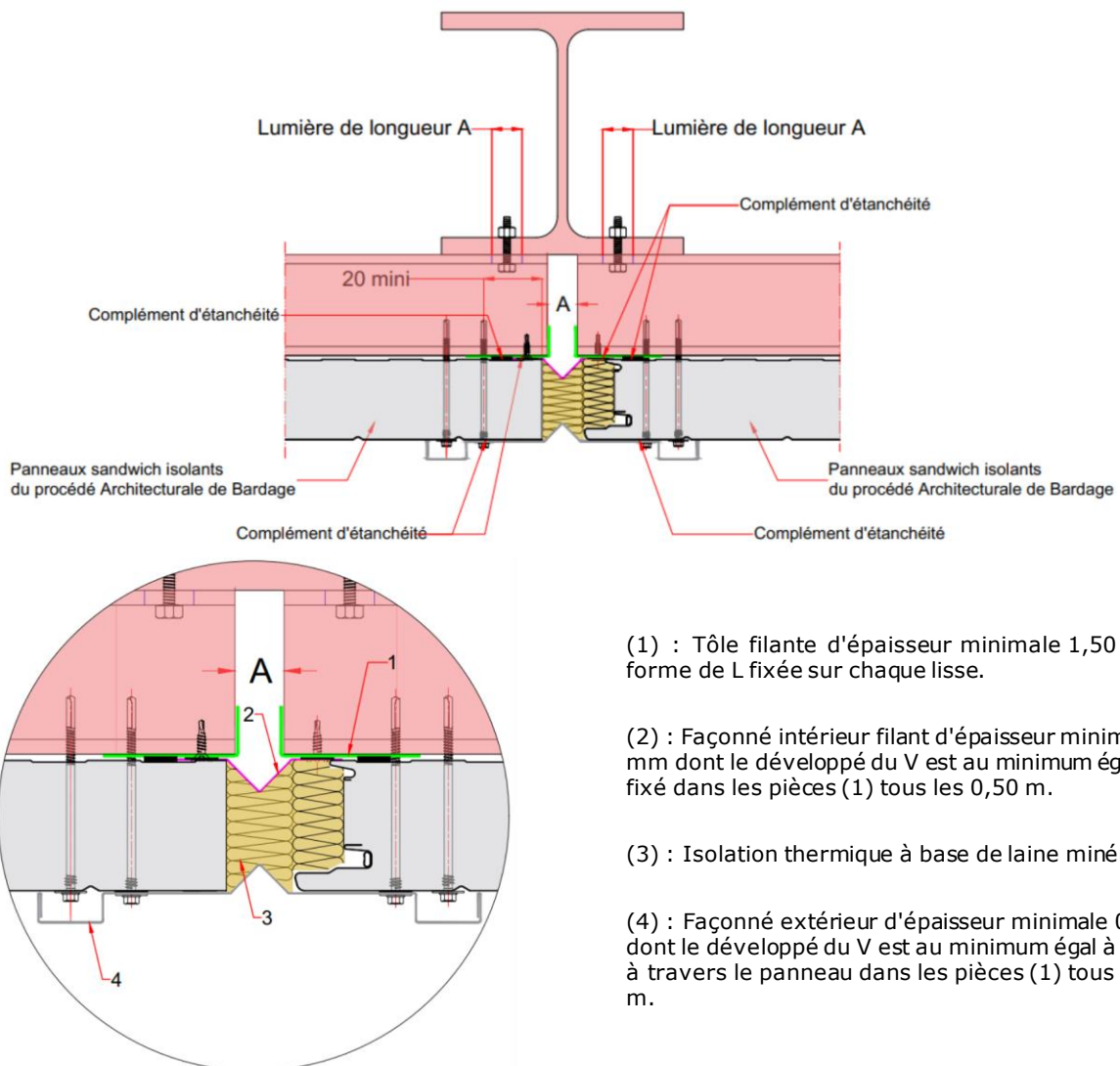
Figure 43 – Exemple d'un joint de dilatation thermique dont le déplacement maximal est de 50 mm en pose verticale
