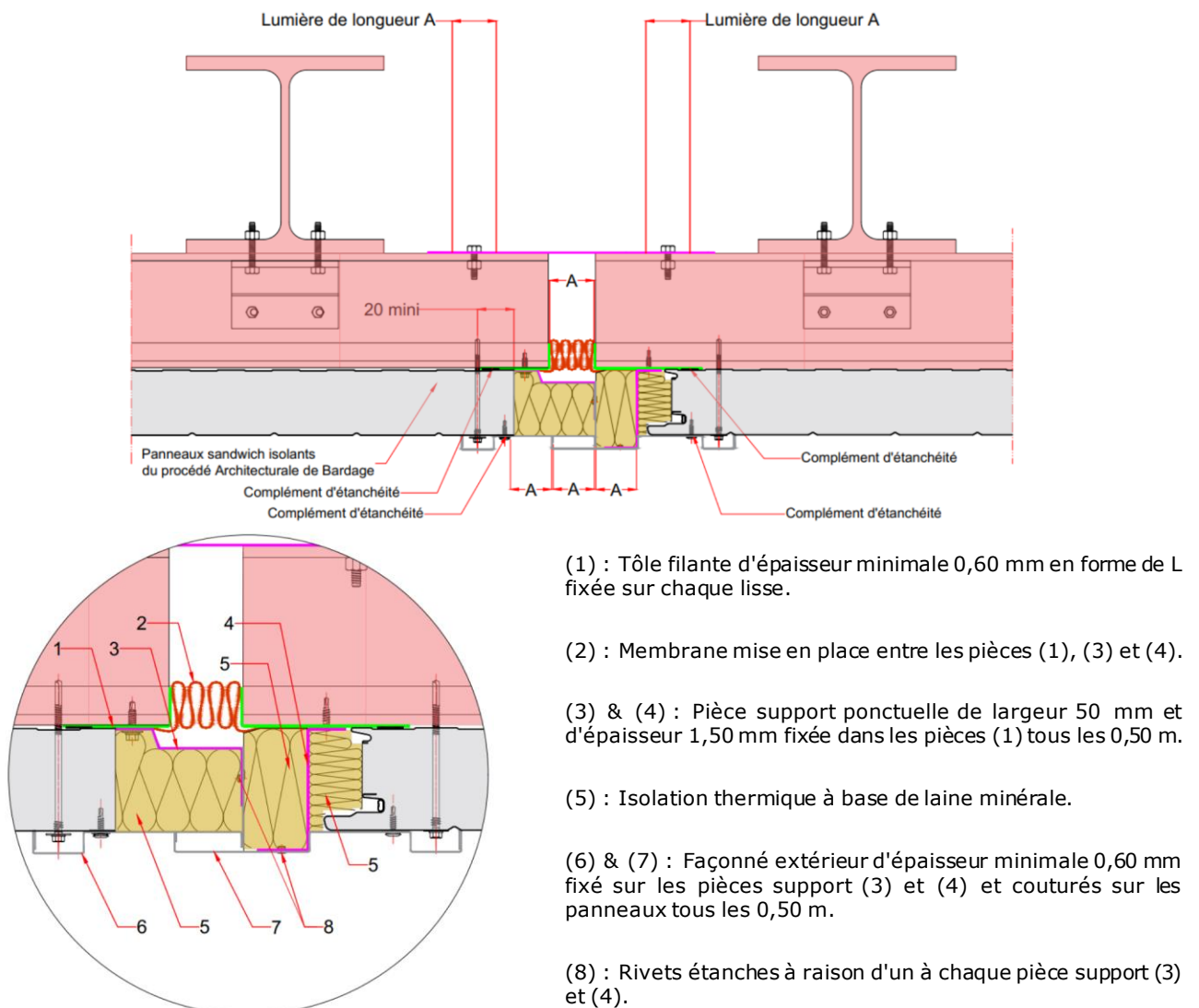
Figure 44 – Exemple d'un joint de dilatation dont le déplacement maximal est de 150 mm en pose verticale
