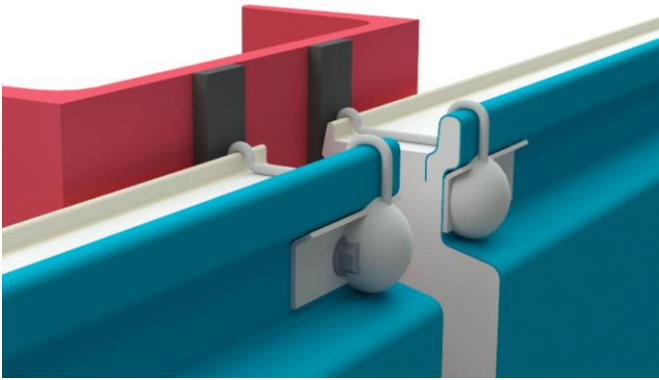
Exemple avec joints mousse 20 x 5 mm disposés sur appuis
