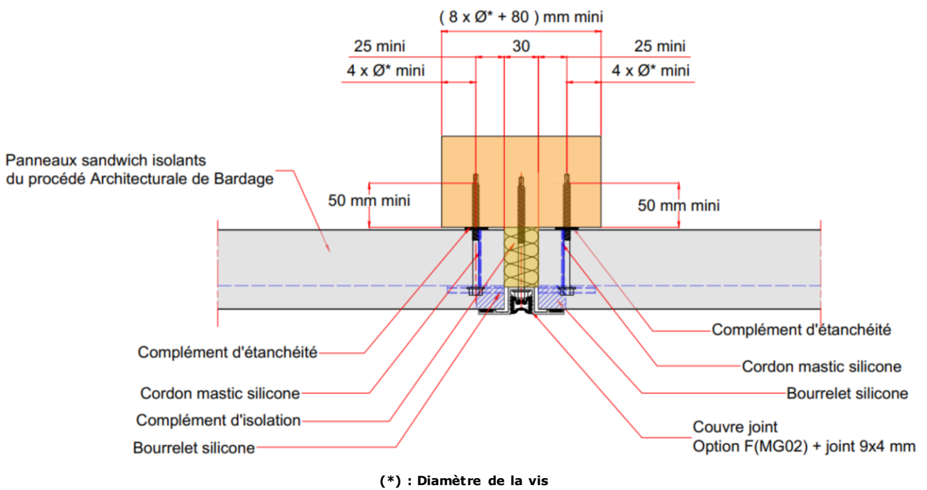
Figure 22 – Exemple d'une jonction verticale en pose horizontale sur ossature bois avec couvre-joint option F (MG02)
