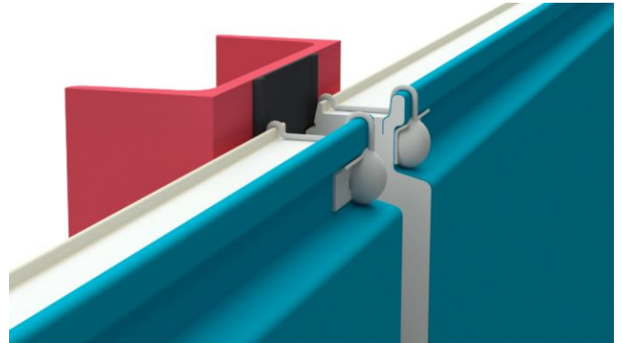
Exemple avec joint EPDM VJ1 ou VJ2 disposé sur appuis
