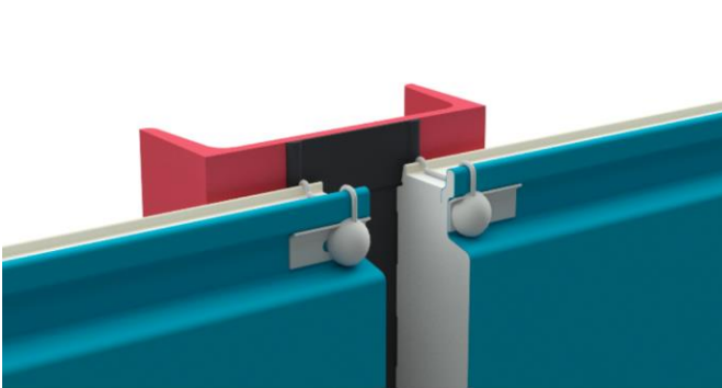
Exemple avec joints mousse 20 x 5 mm disposés sur appuis
