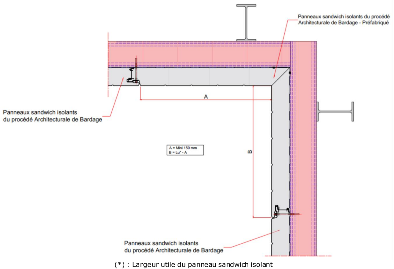
Figure 34 – Exemple d'angle rentrant réalisé avec des panneaux préfabriqués en pose verticale
