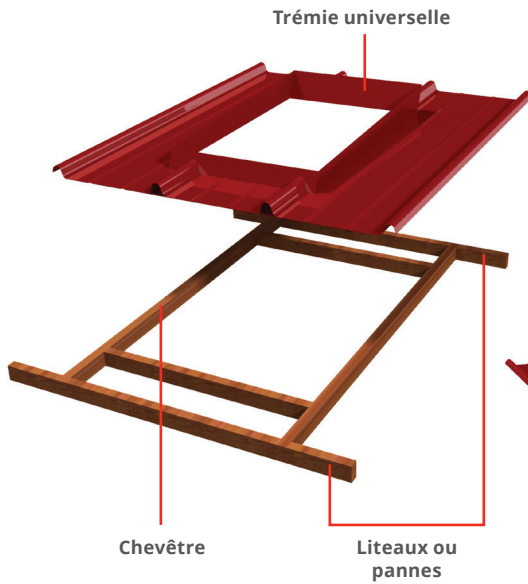
Mise en œuvre du chevêtre
