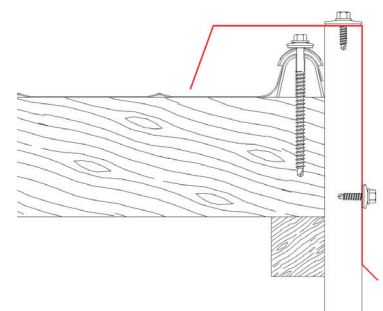
Détails de la fixation de la bande de rive
