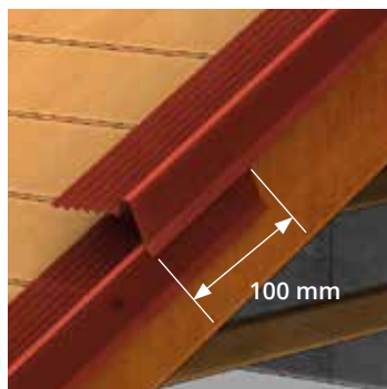
Rive emboîtable sans découpe
