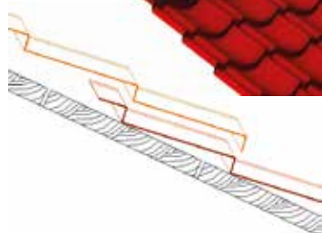
Recouvrement sur 1 tuile
