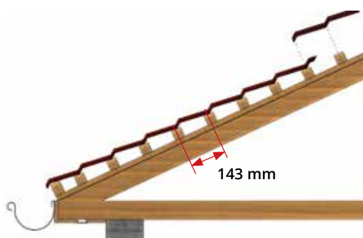
un liteau tous les pureaux
