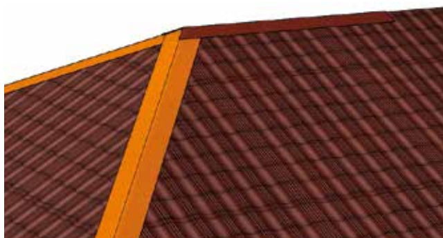
Réalisation de la liaison au faitage
