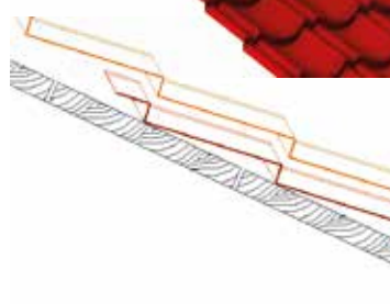
Recouvrement sur 2 tuiles et plus
