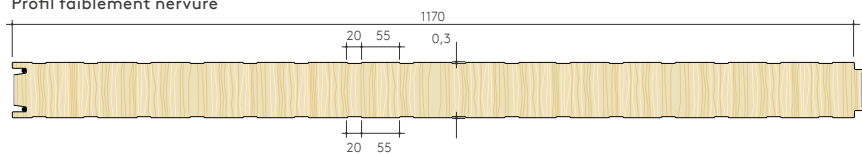
Profil faiblement nervuré
