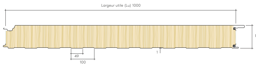
Profil lisse
