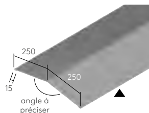
Sous-faîtière
