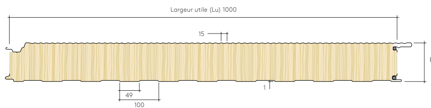
Profil micro-nervuré
