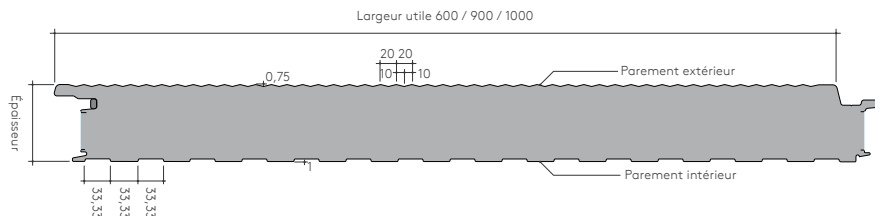
Profil Micro-Rib*
