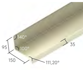
Rive contre mur
